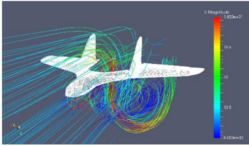
図3 数値流体力学計算(回転翼機モード)
